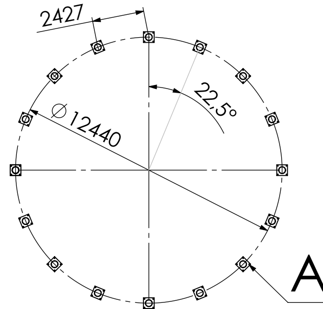
KESIT A-A ÖLÇEK 1 : 180
