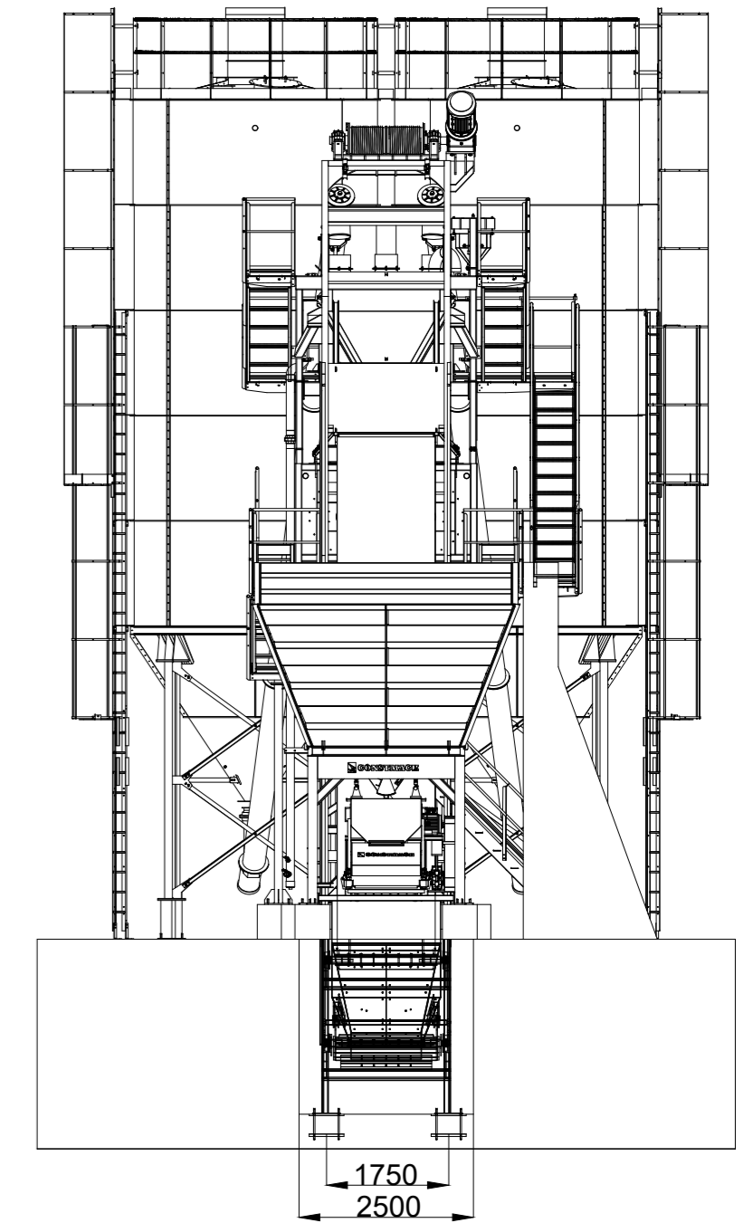
A-A SECTION
