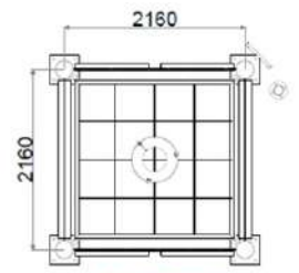
A-A SECTION
