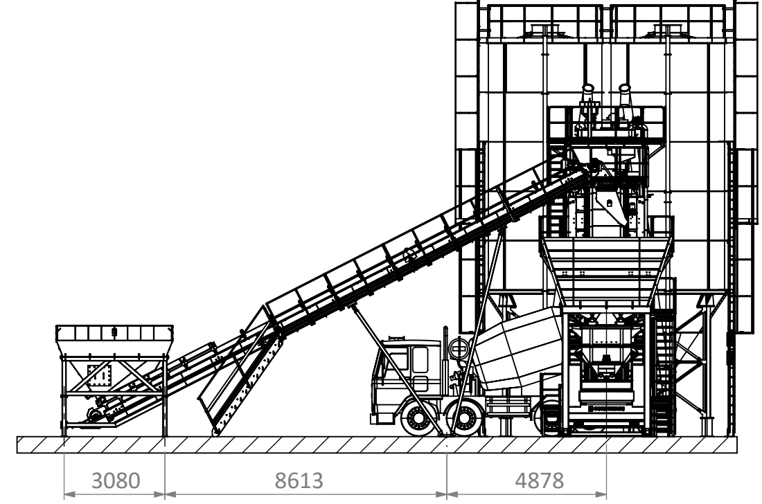
KESIT A-A ÖLÇEK 1 : 160
